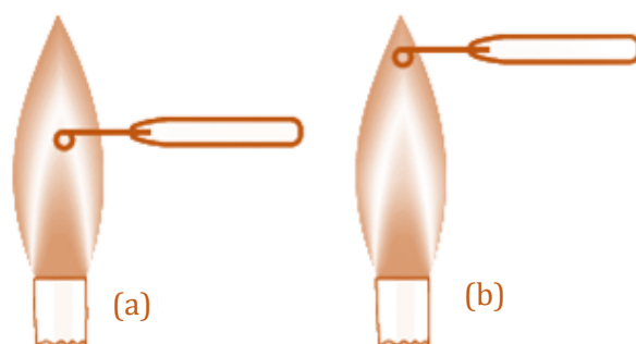
Fig. : Borax bead test
